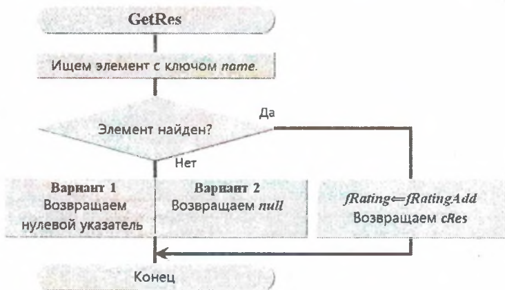
Рис. 3 – Блок-схема метода GetRes класса ResourcesManager
