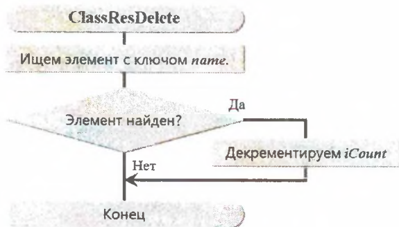
Рис. 4 – Блок-схема метода ClassResDelete класса ResourcesManager
