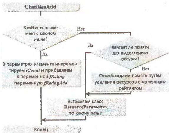
Рис. 2 – Блок-схема метода ClassResAdd класса ResourcesManager
